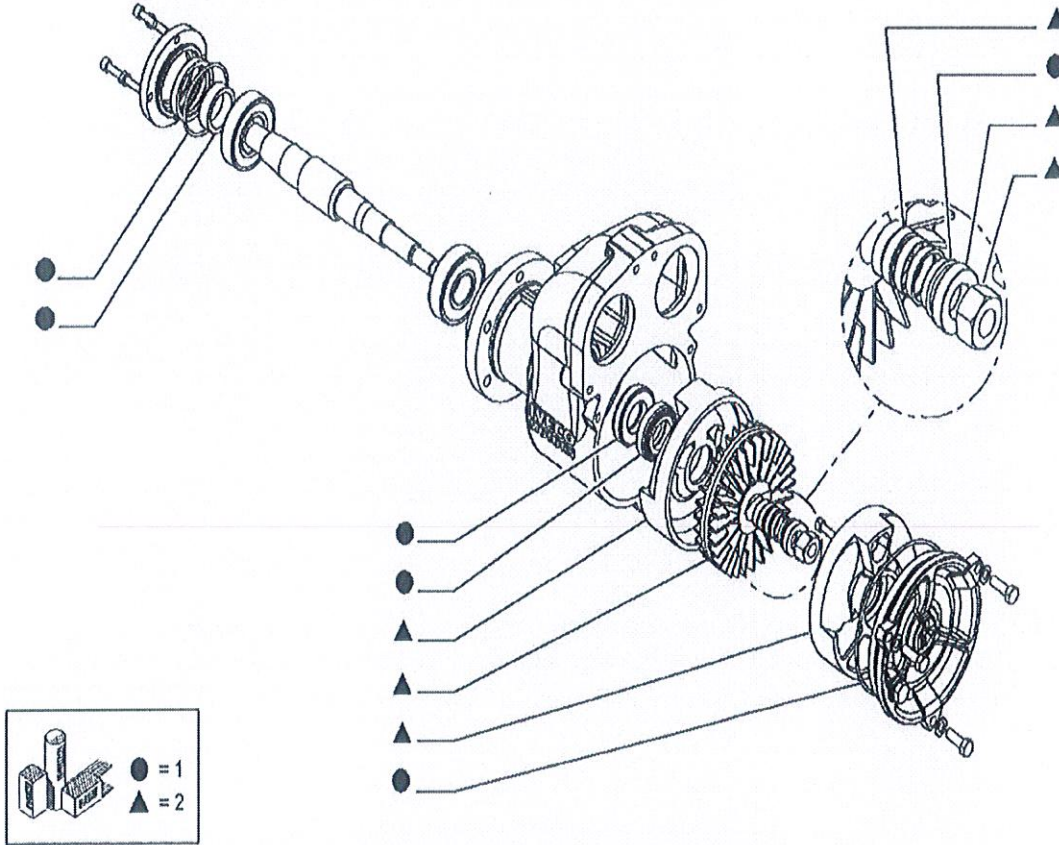
Şekil-1 Deniz Suyu Pompası Parça Resimleri
