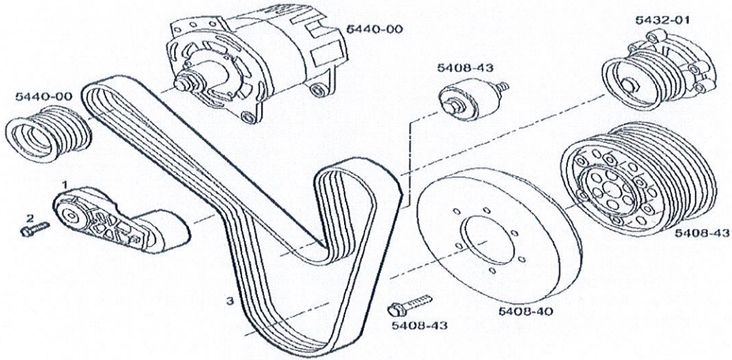
Şekil-3 V-Belt( V-Kayış Resmi)
